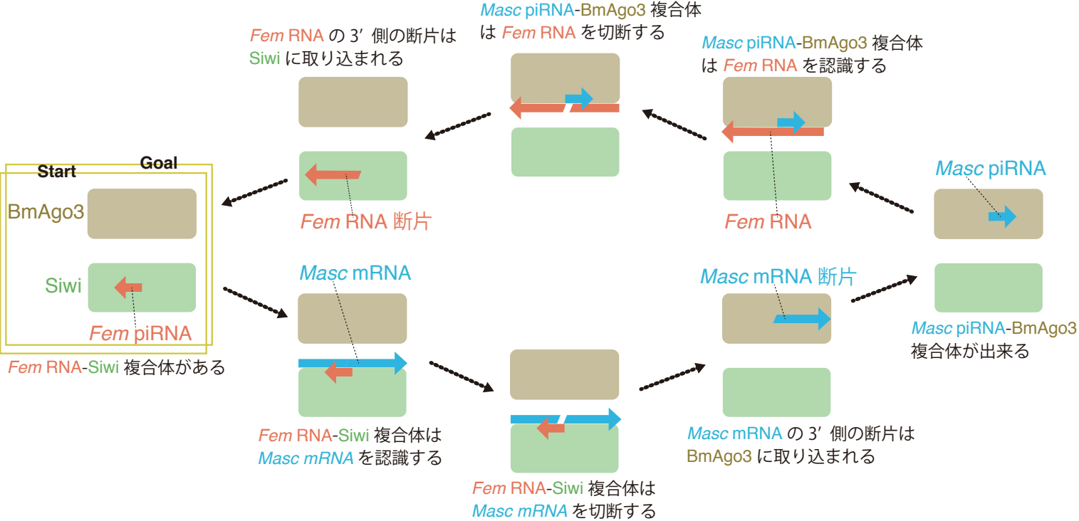
図 1：内在性の ping-pong サイクルの模式図（ Fem piRNA と Masc piRNA を例に）
